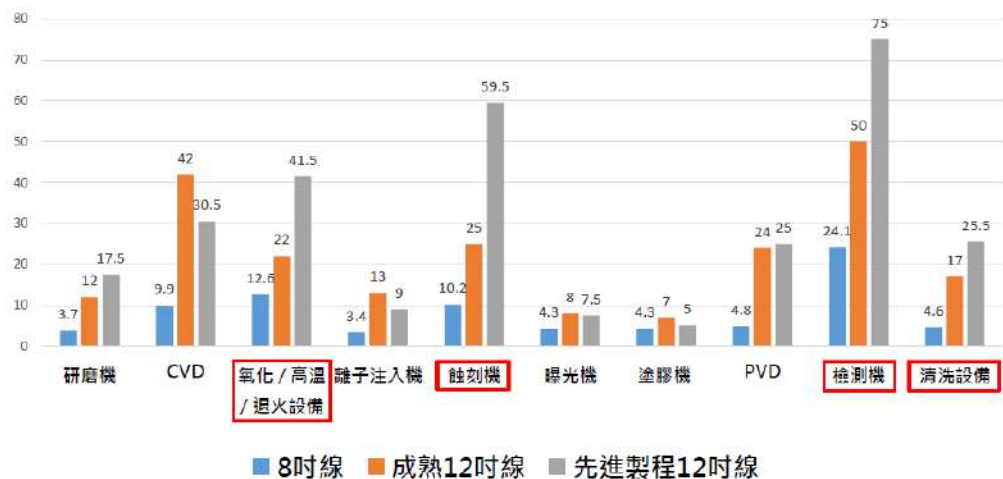
圖三 設備需求量(月產能一萬片)
